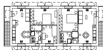
PIANTA PIANO PRIMO "FABBRICATO B"
