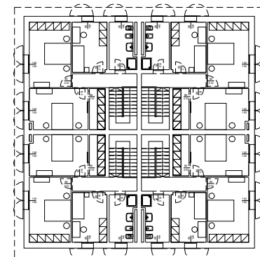
PIANTA PIANO PRIMO "QUADRIFAMILIARE"
