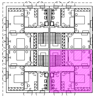
PIANTA PIANO PRIMO "QUADRIFAMILIARE"
