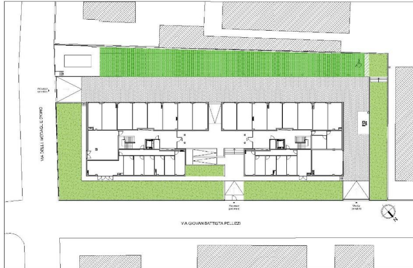
PIANO PRIMO
